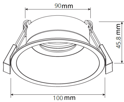
Deep Trim Ø95
